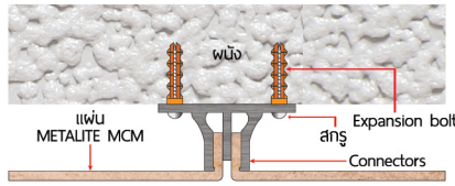
ต่อแบบเว้นร่อง
