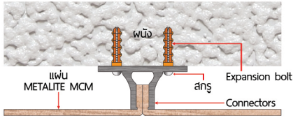
ต่อแบบชนชิด
