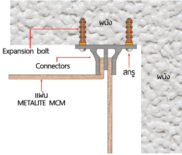
เข้ามุมในแบบเว้นร่อง
