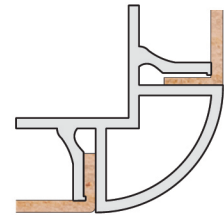
ตัวต่อมุม
