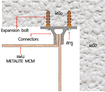
เข้ามุมในแบบชนชิด
