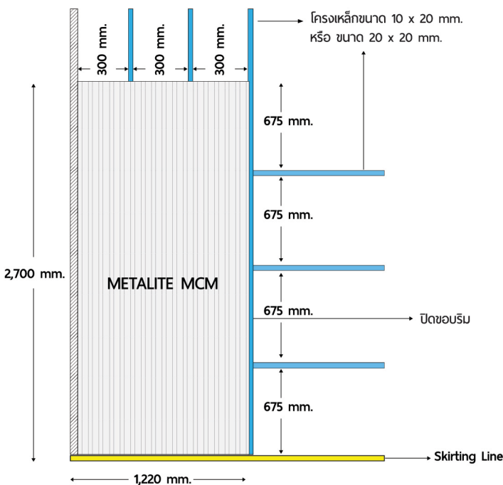
รูปด้านหน้า
